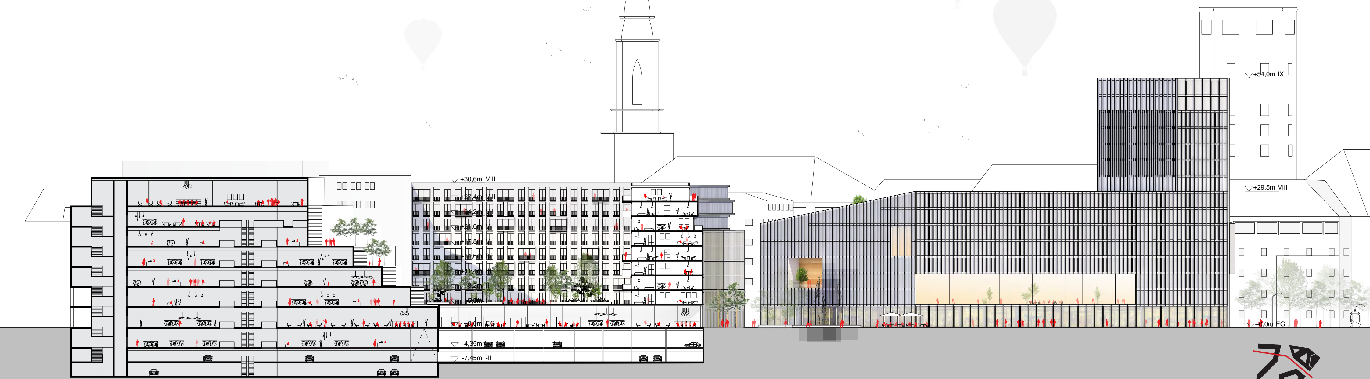
SCHNITT AA 1-500
